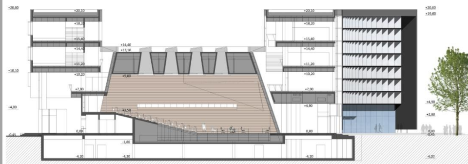
presjek B-B
