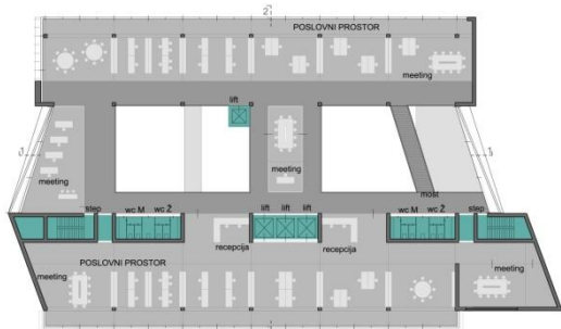
● tlocrt karakterističnog kata / 5 kat 1:200
