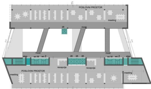
● tlocrt karakterističnog kata / 7 kat 1:200
